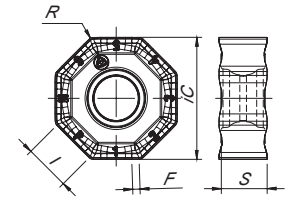
ONH(K)X-MK | LP | MP
